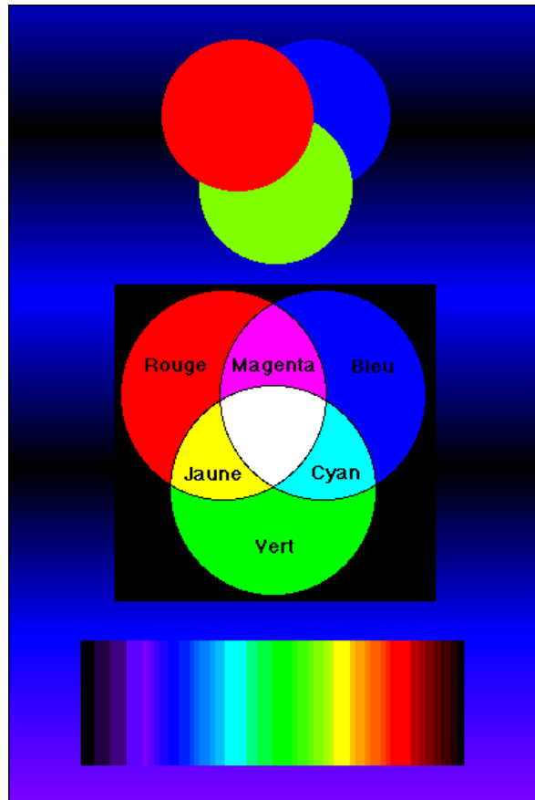
- Spectre des couleurs visibles -
