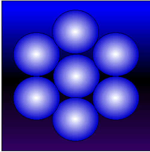
Sept cercles
